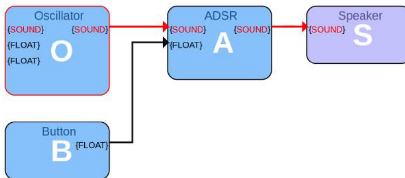
Figura 3: Diagrama do Mosaicode composto por blocos e conexões entre eles.
